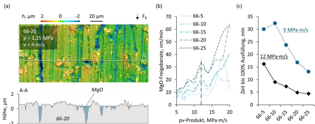
Abbildung 47: Ausfüllung der Furchen durch freigegebenes MgO: (a) Darstellung anhand eines beispielhaften Profilschnitts (66-20, p = 1,25 MPa, v = 4 m/s); (b) MgO-Freigabe- rate abhängig von Belastung und Füllstoffgehalt; (c) Zeit bis zur vollständigen Ausfüllung des Furchenvolumens.
