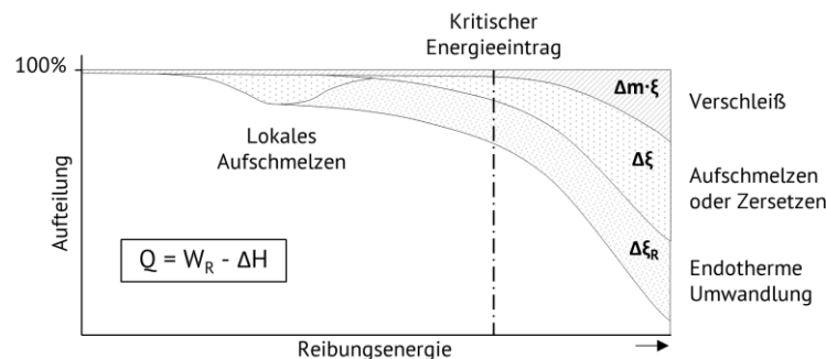
Abbildung 8: Veränderung des energetischen Gleichgewichts in einem Tribosystem mit zunehmender Reibungsenergie durch verschiedene enthalpiebehaftete Stoffänderungen (schematisch).
